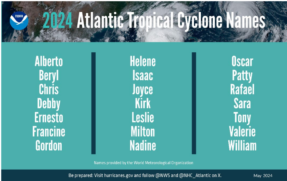
Nòmbernan pa e temporada di orkan 2024 (NOAA).
